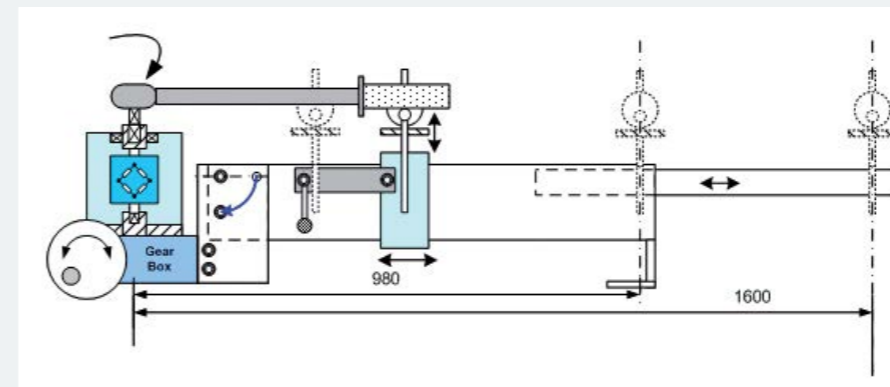
Statische QC-Drehmomentaufnehmer
